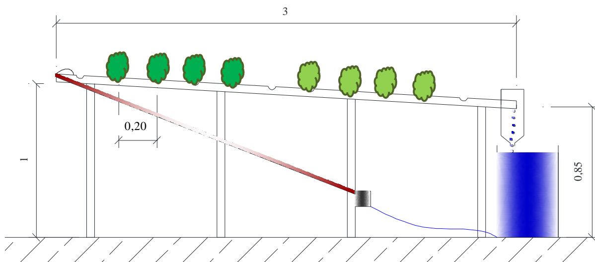
Figura 3 - Perfil do sistema hidropônico.
