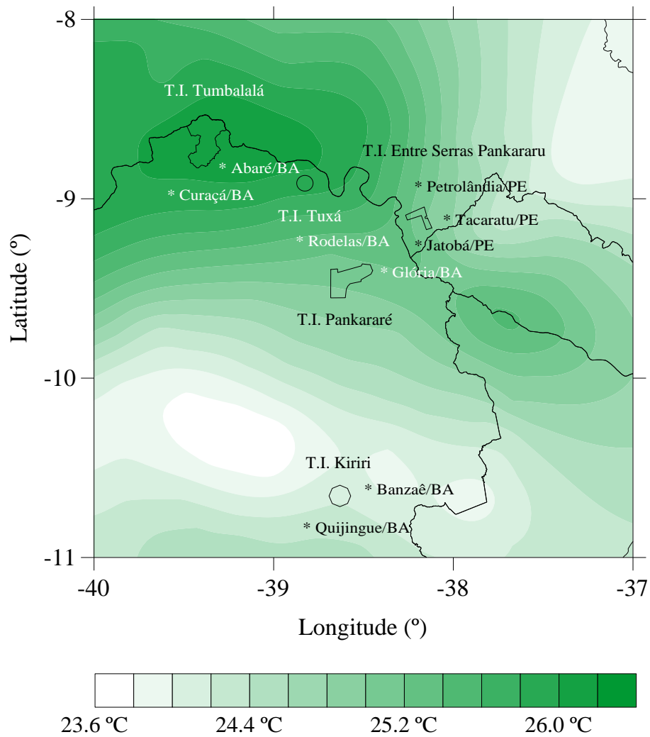
Figura 8. Carta da temperatura média anual para o período de 1911 - 1990
