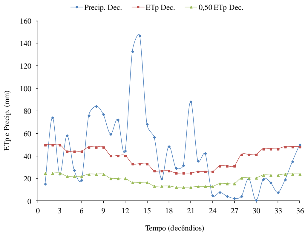
Figura 12. Estação de crescimento de Banzaê/BA – Quijingue/BA, representação com base na acumulação decencial de precipitação pluviométrica e evapotranspiração potencial no cenário chuvoso, no período 1963-1990
