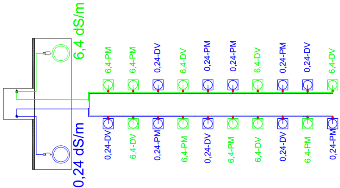
Figura 5. Croqui do arranjo experimental.
