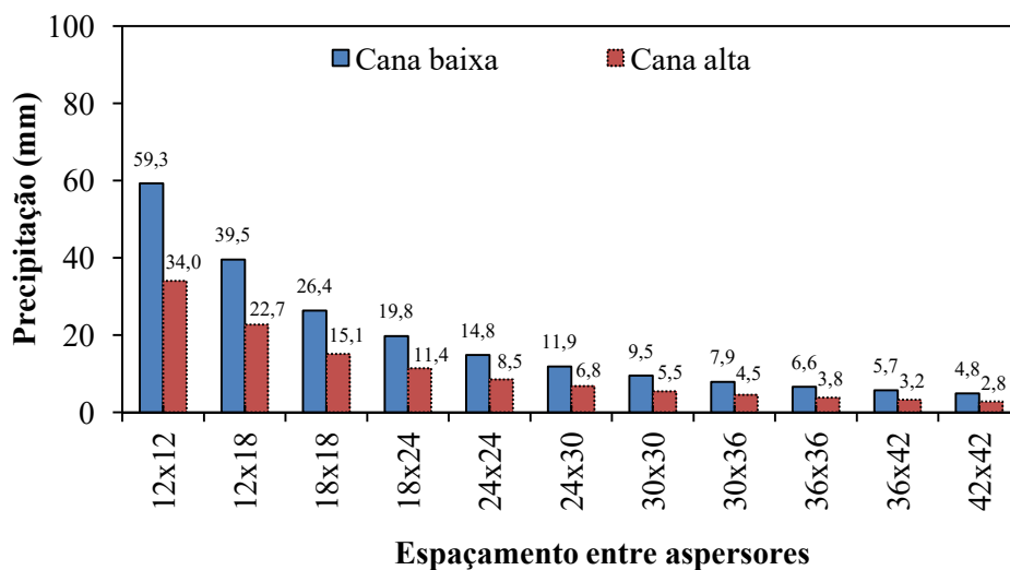
Figura 19. Média de lâmina precipitada para cana baixa e cana alta nos diferentes espaçamentos entre aspersores.
