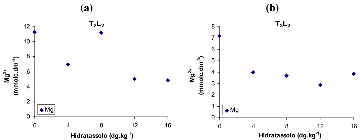
Figura 2C (a;b): Diagramas de dispersão dos dados médios observados da variável Mg nas épocas de balanço hídrico ( T_2 , T_3 ), em função das doses de hidratassolo (H), fixando-se a lâmina de irrigação ( L_2 ).
