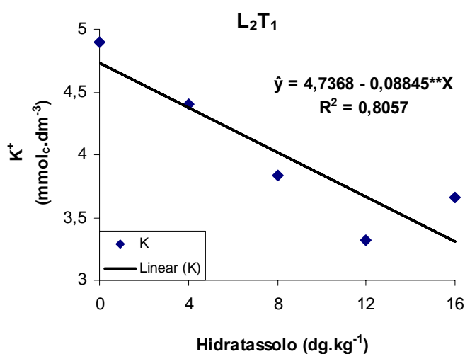
Figura 12 - Concentração de potássio (K) em função da variação crescente de doses de hidratassolo (H), fixando-se a lâmina de irrigação (L 2 ), na primeira época de observação (T 1 ).
