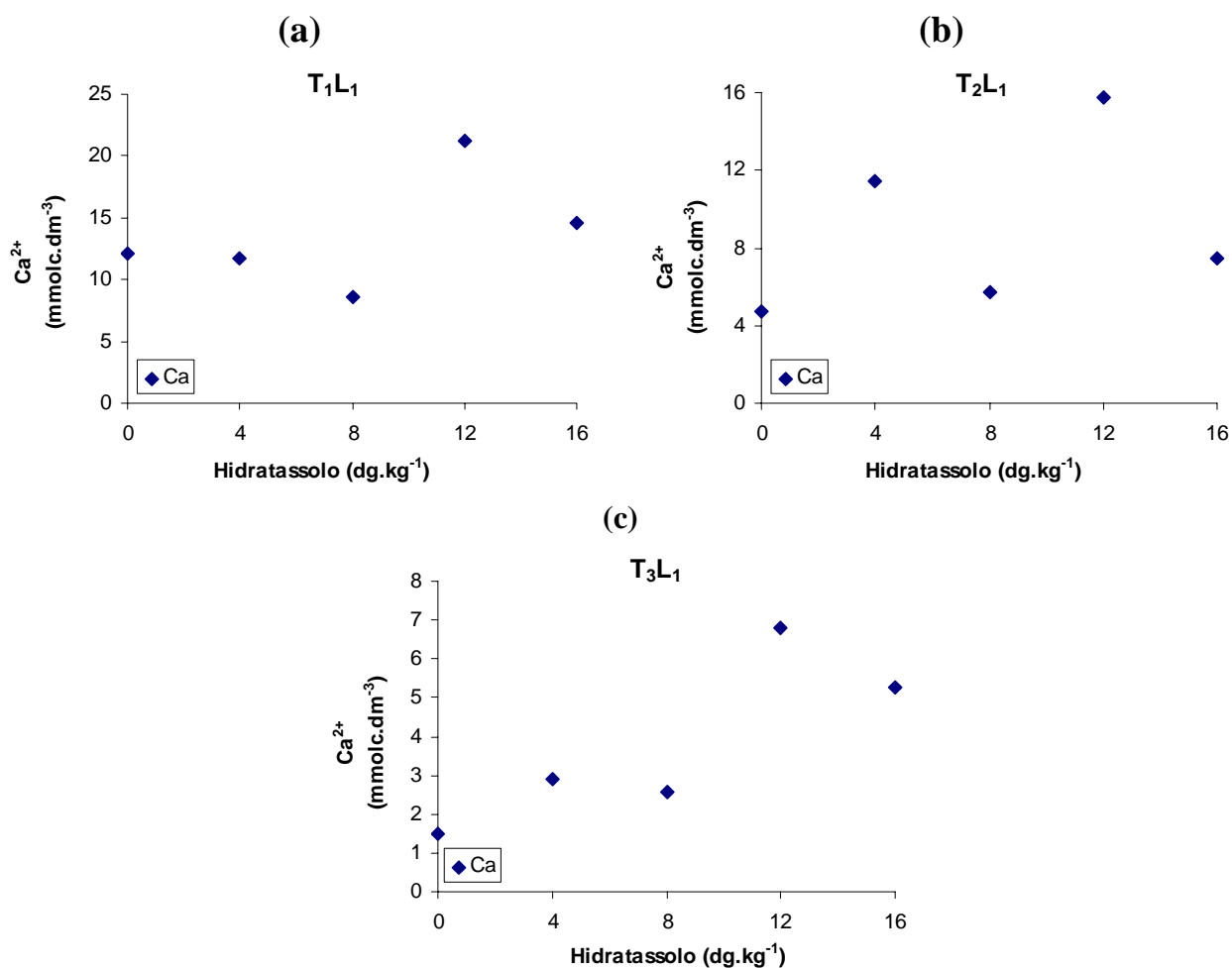
Figura 1B (a,b,c): Diagramas de dispersão dos dados médios observados da variável Ca nas épocas de balanço hídrico (T 1 , T 2 , T 3 ), em função das doses de hidratassolo (H), fixando-se a lâmina de irrigação (L 1 ).
