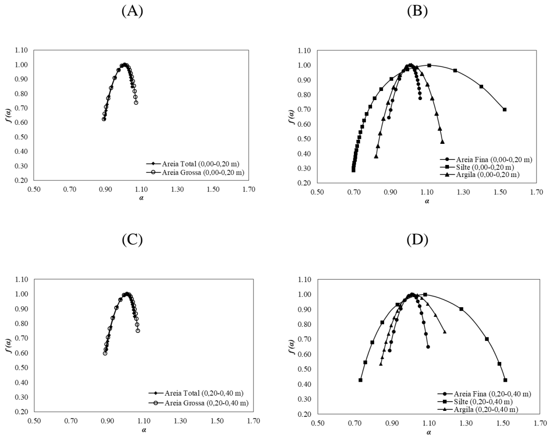
Figura 9. Espectros multifractal para as frações granulométricas do solo quantificadas pelo método do densímetro: areia total e areia grossa, na camada de 0,00-0,20 m (A), areia fina, silte e argila, na camada de 0,00-0,20 m (B), areia total e areia grossa, na camada de 0,20-0,40 m (C) e areia fina, silte e argila, na camada de 0,20-0,40 m (D), para momentos estatísticos da ordem q+ , 10, q- , 10.
