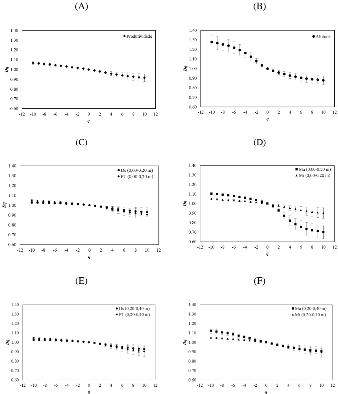
Figura 3. Espectros de dimensão generalizada, D_q versus q , em incrementos de -1,0 de q , para a produtividade da cana-de-açúcar (A), altitude (B) e atributos físicos do solo nas camadas de 0,00-0,20 e 0,20-0,40 m (C), (D), (E) e (F).
