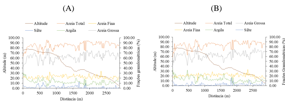
Figura 8. Distribuição espacial das frações granulométricas do solo pelo método do densímetro para as camadas de 0,00-0,20 m (A) e 0,20-0,40 m (B) ao longo dos 145 pontos de amostragem.
