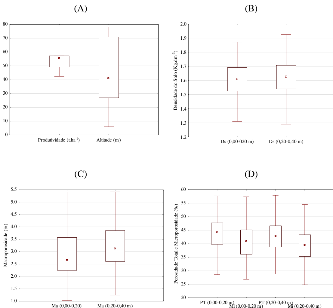
Figura 5. Gráficos “box plot” da altitude e produtividade da cana-de-açúcar (A); densidade do solo (B), macroporosidade (C), porosidade total e microporosidade (D), nas camadas de 0,00-0,20 e 0,20-0,40 m ao longo do transecto do estudo.
