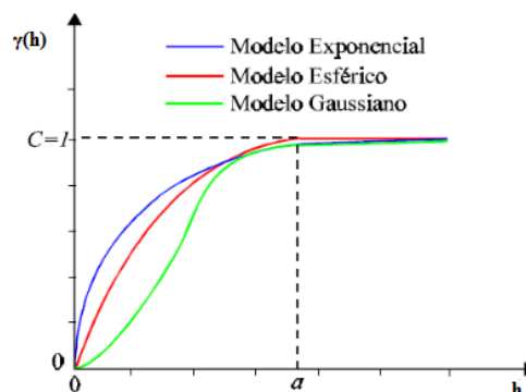
Figura 2. Modelos de semivariogramas escalonados.
