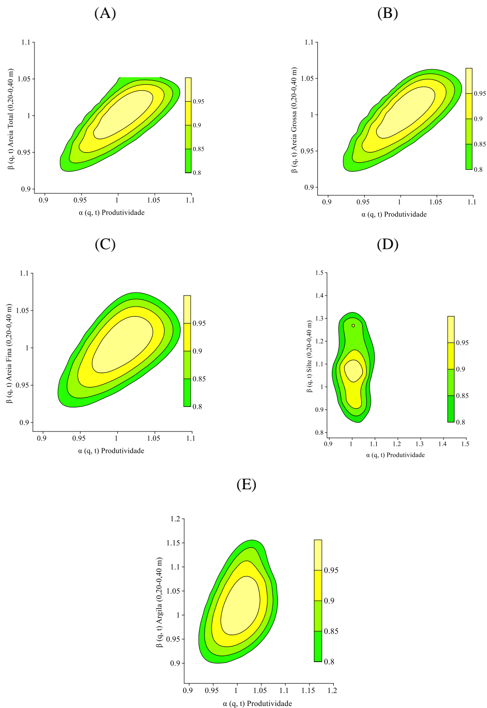
Figura 2. Espectros multifractais da distribuição conjunta da produtividade da cana-de-açúcar (eixo horizontal) e frações granulométricas do solo quantificadas pelo método do densímetro (eixo vertical), na camada de 0,20-0,40 m, nomeados areia total (A), areia grossa (B), areia fina (C), silte (D) e argila (E). Diferentes cores mostram a dimensão conjunta dos dois índices de escala: \alpha(q, t) e \beta(q, t) .
