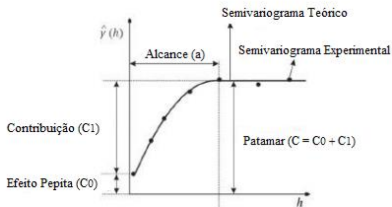
Figura 1. Esquema de semivariograma e seus parâmetros.
