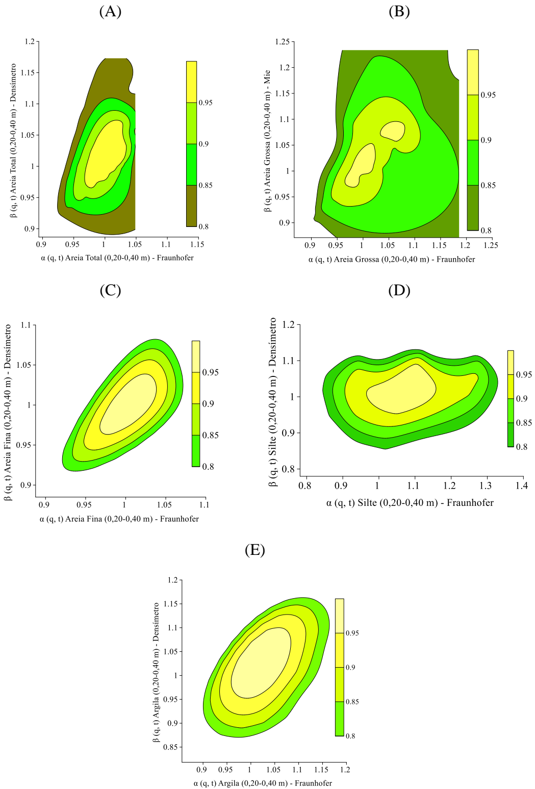
Figura 18. Espectros multifractais da distribuição conjunta das frações granulométricas do solo quantificadas pelos métodos de difração a laser de Fraunhofer (eixo horizontal) e do densímetro (eixo vertical), na camada de 0,20-0,40 m, nomeados areia total (A), areia grossa (B), areia fina (C), silte (D) e argila (E). Diferentes cores mostram a dimensão conjunta dos dois índices de escala: \alpha(q, t) e \beta(q, t) .
