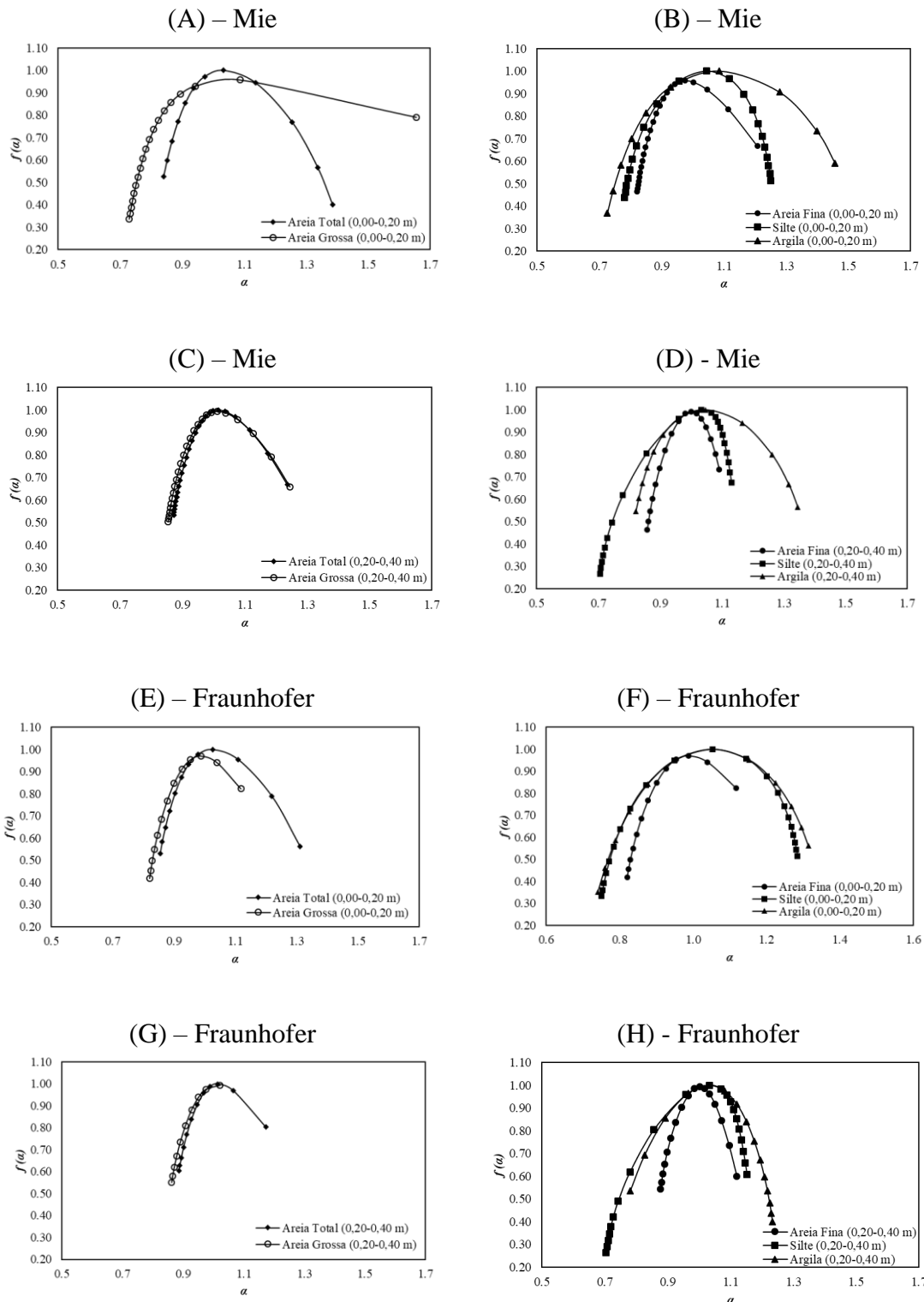
Figura 10. Espectros multifractais para as frações granulométricas do solo quantificadas pelo método de difração a laser: de Mie - areia total e areia grossa, na camada de 0,00-0,20 m (A), areia fina, silte e argila, na camada de 0,00-0,20 m (B), areia total e areia grossa, na camada de 0,20-0,40 m (C) e areia fina, silte e argila, na camada de 0,20-0,40 m (D); e de Fraunhofer - areia total e areia grossa, na camada de 0,00-0,20 m (E), areia fina, silte e argila, na camada de 0,00-0,20 m (F), areia total e areia grossa, na camada de 0,20-0,40 m (G) e areia fina, silte e argila, na camada de 0,20-0,40 m (H), para momentos estatísticos da ordem q+ , q- , 10.
