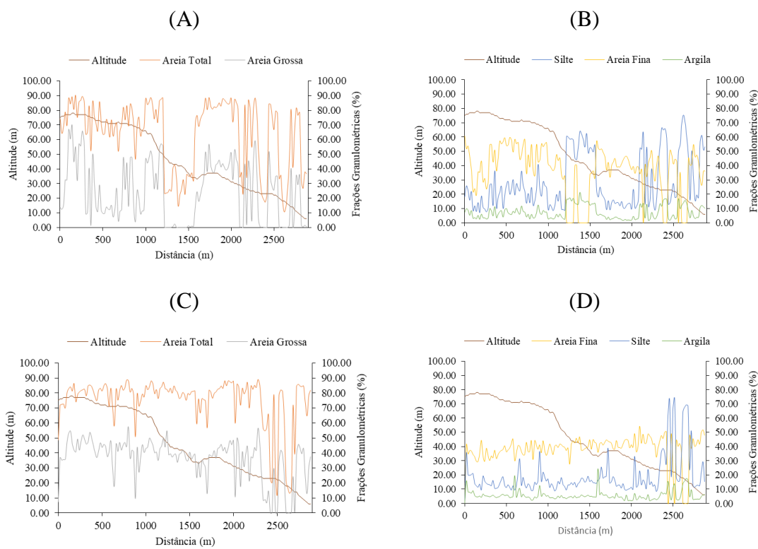
Figura 10. Distribuição espacial das frações granulométricas do solo pelo método de difração a laser de Fraunhofer para as camadas de 0,00-0,20 m (A) e (B) e 0,20-0,40 m (C) e (D) ao longo dos 145 pontos de amostragem.
