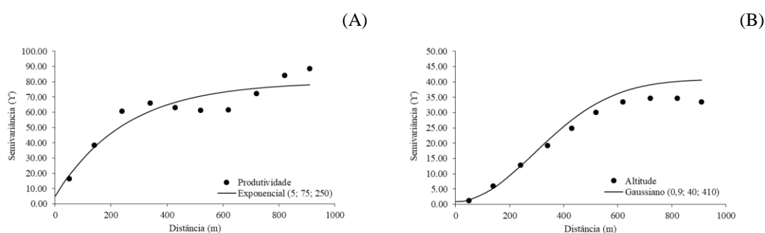
Figura 11. Semivariogramas ajustados para a produtividade da cana-de-açúcar (A) e altitude (B) ao longo do transecto.
