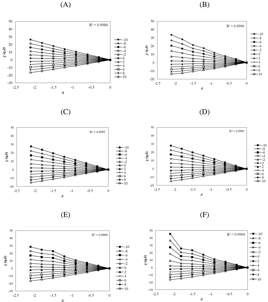
Figura 5. Gráficos log-log da função de partição \chi(q, \delta) em função da escala ( \delta ) em momentos diferentes, q [-10, 10], com incrementos de 1, para a argila, na camada de 0,00-0,20 m (A) e o silte, na camada de 0,20-0,40 m (B), pelo método do densímetro; Para o silte, na camada de 0,00-0,20, pela difração de Mie (C) e Fraunhofer (D); e para a areia grossa, na camada de 0,20-0,40 m, pela difração de Mie (E) e Fraunhofer (F) ao longo do transecto do estudo.
