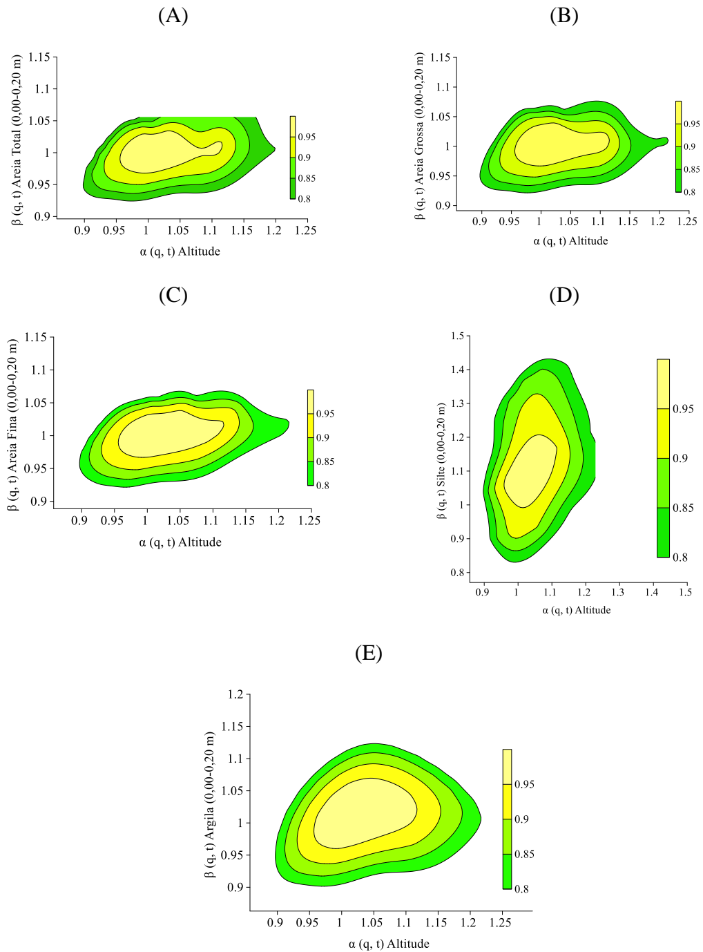
Figura 3. Espectros multifractais da distribuição conjunta da altitude (eixo horizontal) e frações granulométricas do solo quantificadas pelo método do densímetro (eixo vertical), na camada de 0,00-0,20 m, nomeados areia total (A), areia grossa (B), areia fina (C), silte (D) e argila (E). Diferentes cores mostram a dimensão conjunta dos dois índices de escala: \alpha(q, t) e \beta(q, t) .
