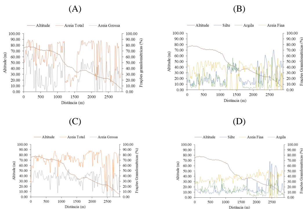
Figura 9. Distribuição espacial das frações granulométricas do solo pelo método de difração a laser de Mie para as camadas de 0,00-0,20 m (A) e (B) e 0,20-0,40 m (C) e (D) ao longo dos 145 pontos de amostragem.
