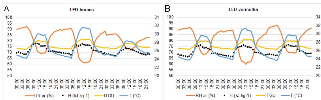
Figura 3. Caracterização térmica do ambiente para os tratamentos T1 (LED vermelha) e T2 (LED branca).
