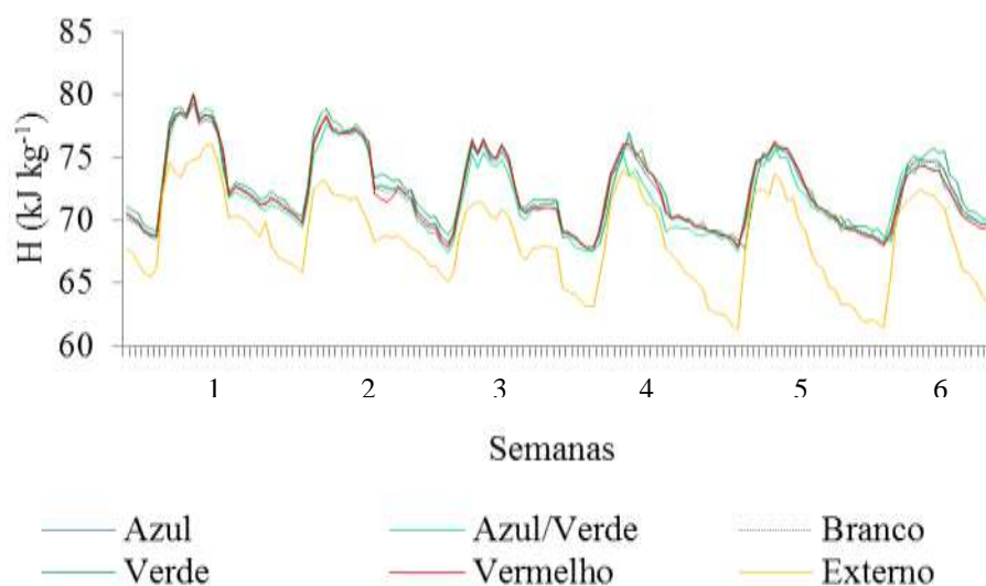
Figura 16 – Variação média horária semanal da entalpia específica (H) no interior e exterior da instalação experimental.
